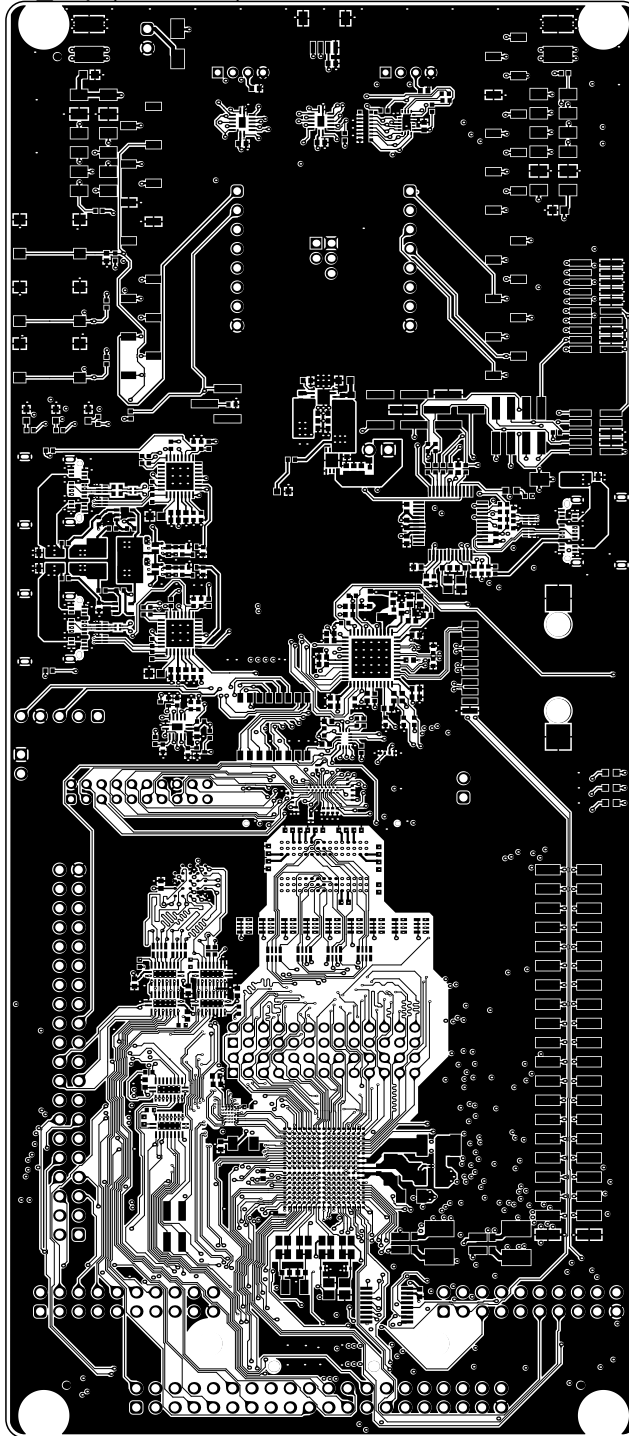
L1 Top (Scale 1:1)
